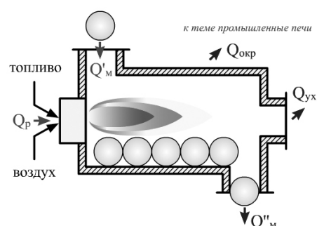
Рис. 1. Схема нагревательной печи к расчету теплового баланса
