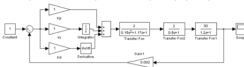
рис.1 Структурная схема
